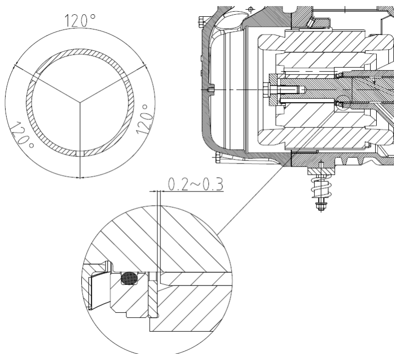
Рисунок 4-8 Схематическая диаграмма втулки со стороны двигателя
