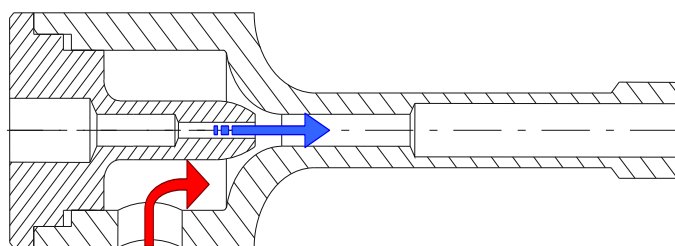
Рисунок 2-22 Эжектор Вентури, вид профиля
