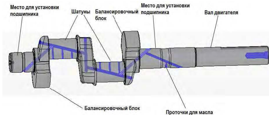
(a) Принципиальная схема коленчатого вала серии SBC
