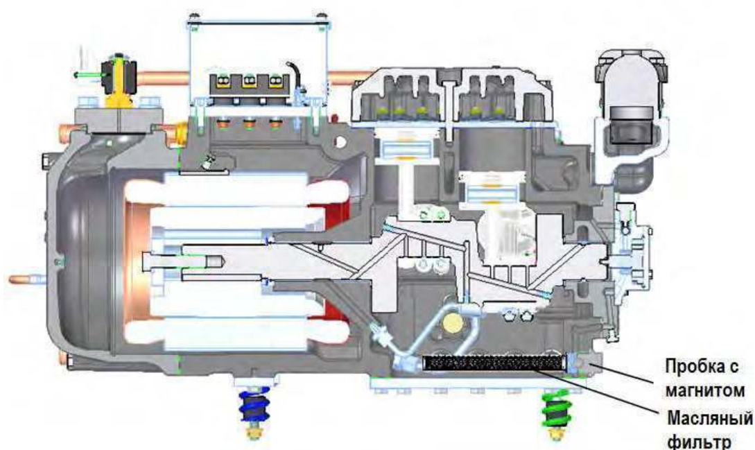
Рисунок 2-6 Масляный фильтр серии SBC
