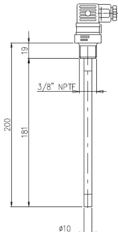
Рисунок 2-9 Габаритные размеры подогревателя картера
