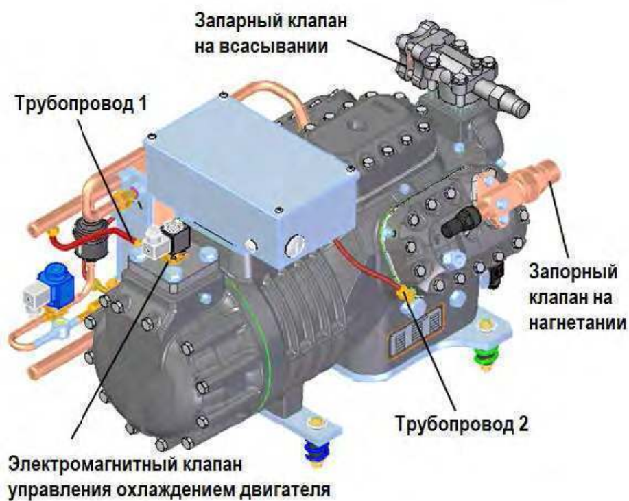
Рисунок 3-3 Схема трубопровода комплекта расширительного клапана с переохладителем жидкости
