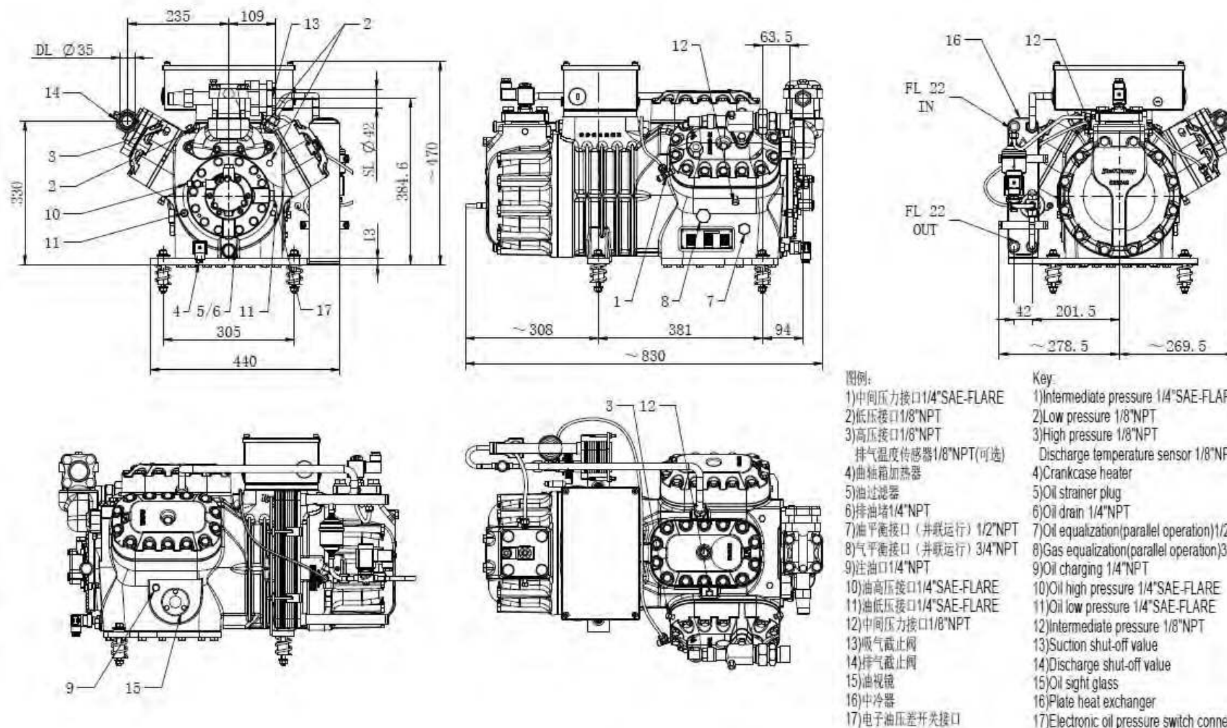
Рисунок 8-2 Габаритные размеры модели SB6C-1600~3000
