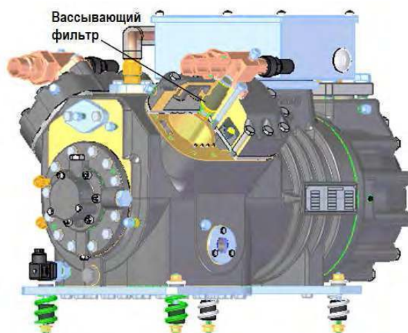
Рисунок 4-1 Расположение всасывающего фильтра серии SB4C
