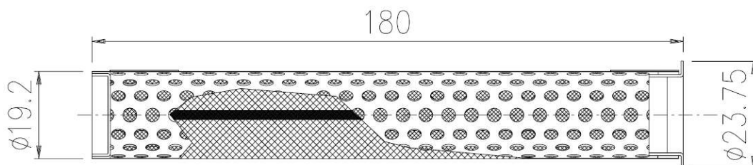
Рисунок 2-7 Масляный фильтр серии SBC
