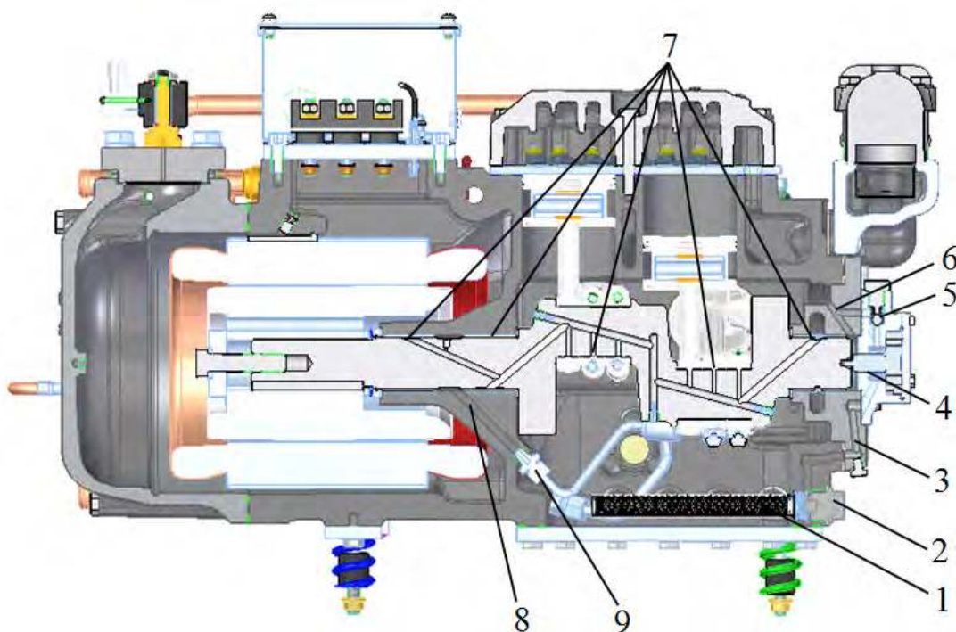
(а) Вид в разрезе компрессоров серии SBC с принудительной смазкой
