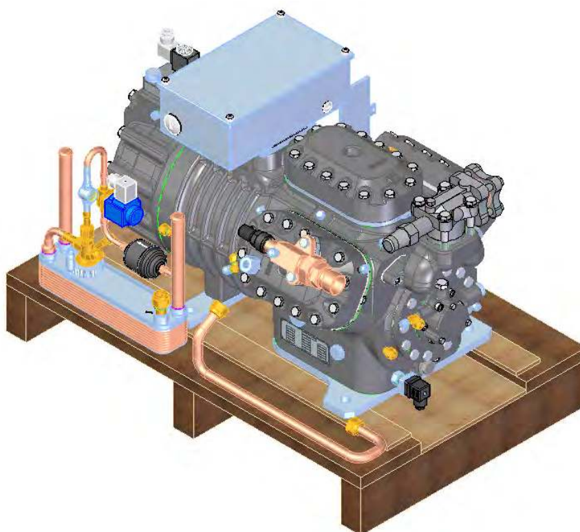
Рисунок 8-4 Схематическая диаграмма расположения компрессора серии SBC
