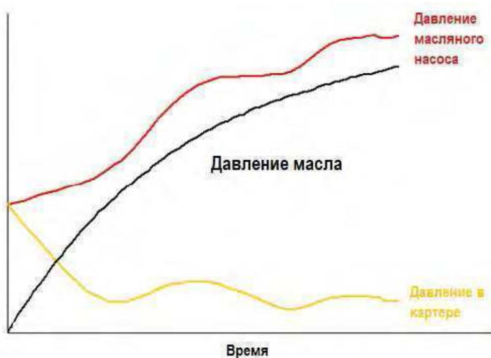
Рисунок 2-4 Перепад давления масла – временная диаграмма во время запуска компрессора
