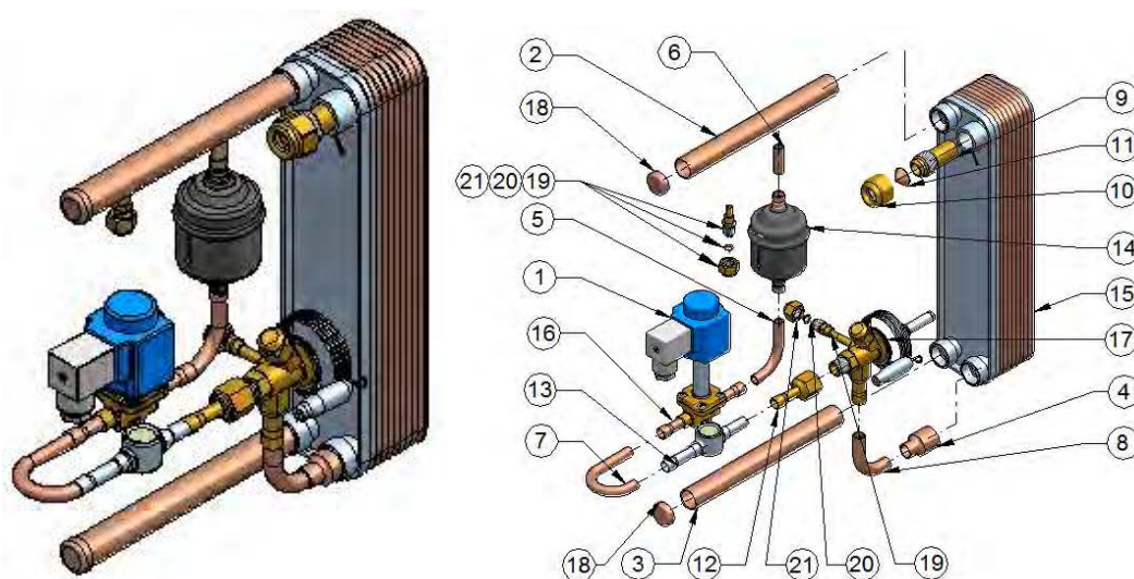
Рисунок 3-1 Схема комплекта расширительного клапана с переохладителем жидкости
