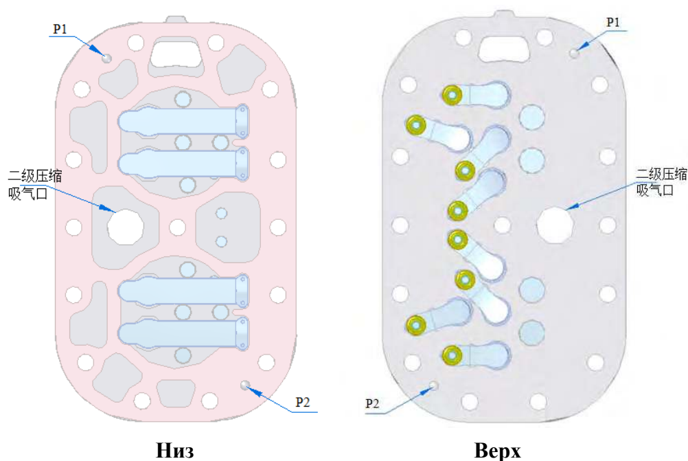
(б) Схематическая диаграмма тарелки клапана сжатия второй ступени
