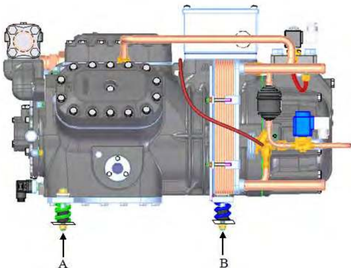
Рисунок 8-7 Положение сборки пружинного амортизатора компрессора серии SBC
