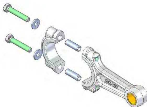
Рисунок 4-5 Схематическая диаграмма компонентов шатуна серии SBC
