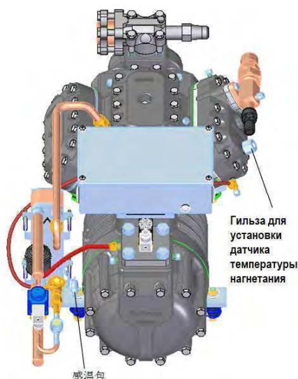
Рисунок 3-2 Комплект расширительного клапана с переохладителем жидкости
