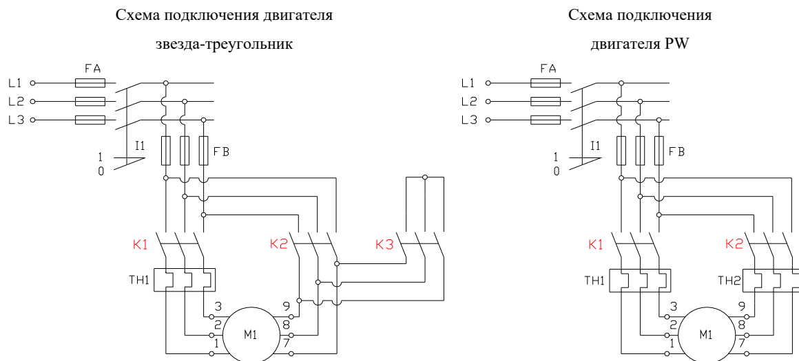
Рисунок 5-3 (а) Схема подключения двигателя звезда-треугольник и двигателя с частичной обмоткой
