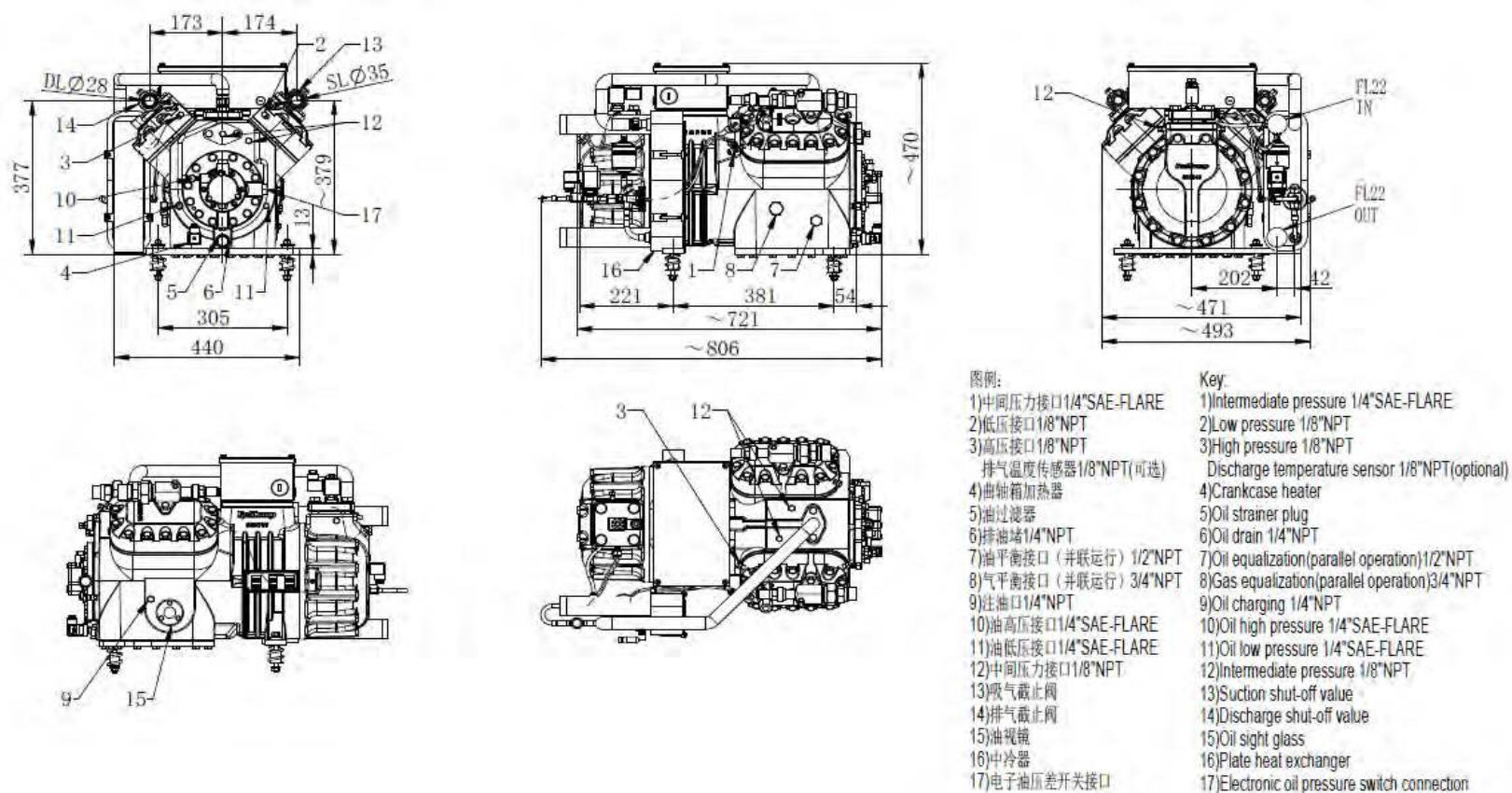
Рисунок 8-1 Габаритные размеры модели SB4C-1200/1400
