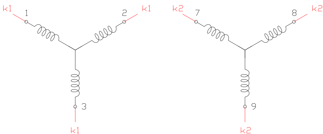
Катушка двигателя
