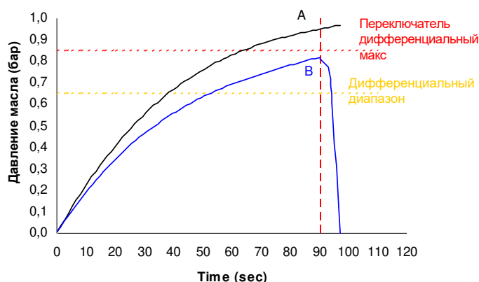
Рисунок 2-12 Фаза запуска переключателя перепада давления масла
