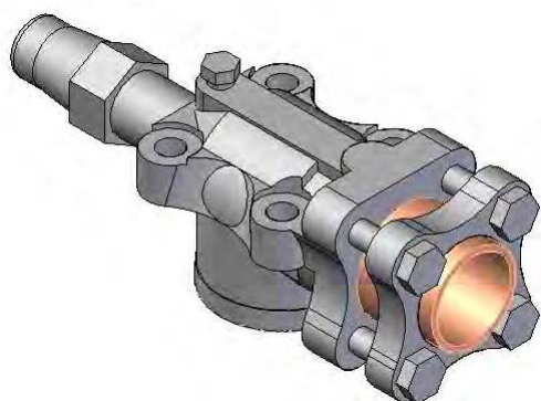
(a) Всасывающий запорный клапан
