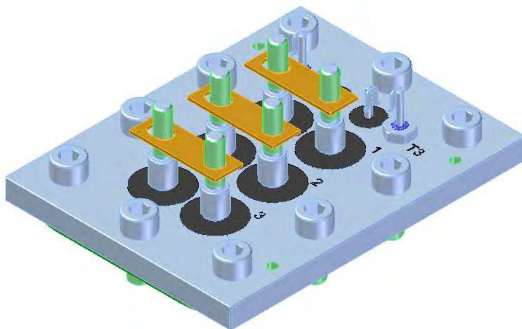
Рисунок 5-6 Схема подключения DOL
