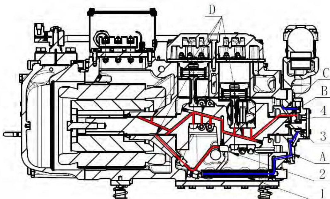
(b) Принципиальная схема принудительной смазки серии SBC
