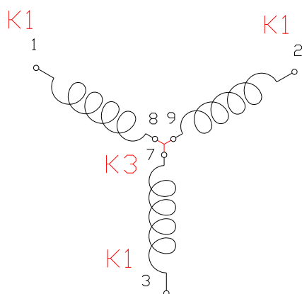
Соединение звездой
