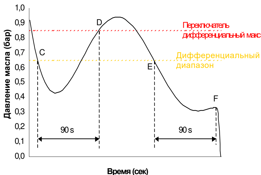
Рисунок 2-13 Этапы работы реле перепада давления масла
