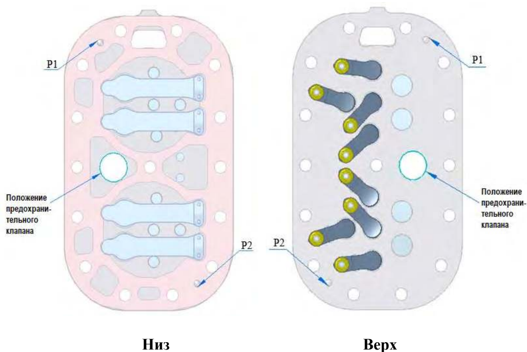
(а) Схематическая диаграмма клапанной доски сжатия первой ступени
