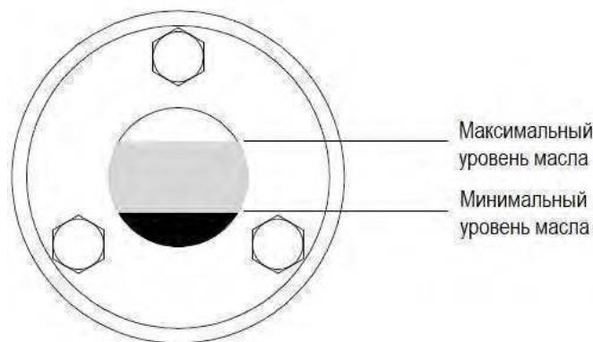
Рисунок 12-1 Диапазон уровня масла
