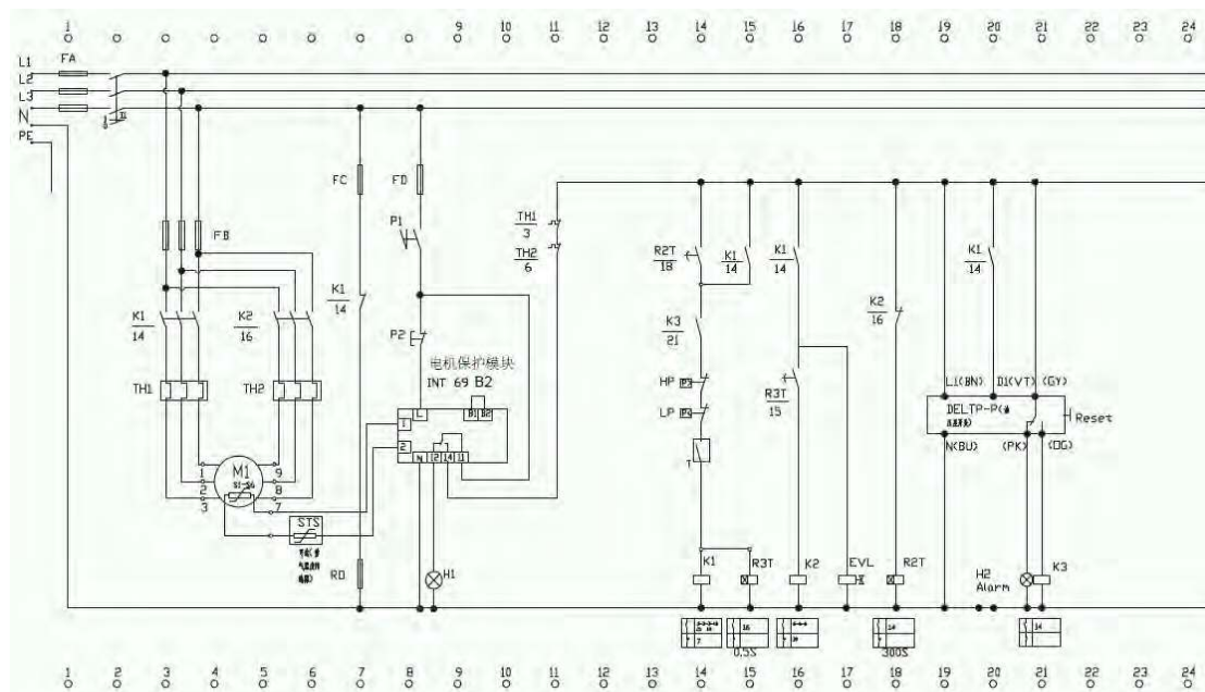
Рисунок 2-16 Электрическая схема электронного реле перепада давления масла
