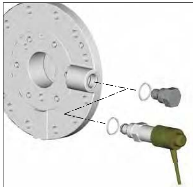
Рисунок 2-17 Схема установки электронного реле перепада давления масла
