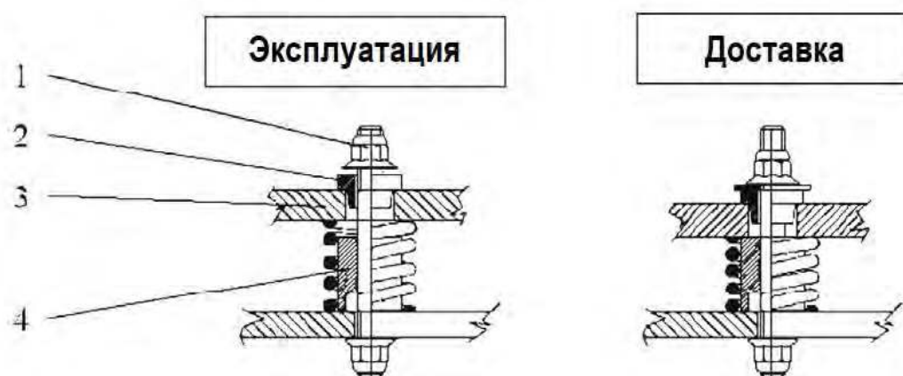
Рис. 8-8 Различные положения пружины во время эксплуатации и транспортировки компрессора
