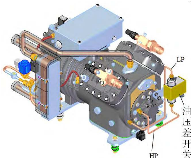
Рисунок 2-18 Схема установки механического реле перепада давления масла MP54
