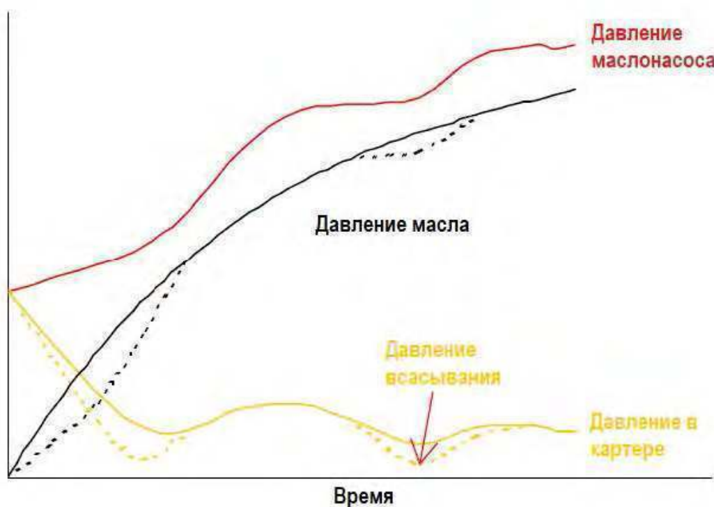
Рисунок 2-5 Кривая зависимости давления масла от времени между всасывающей частью и картером, оборудованным обратным клапаном
