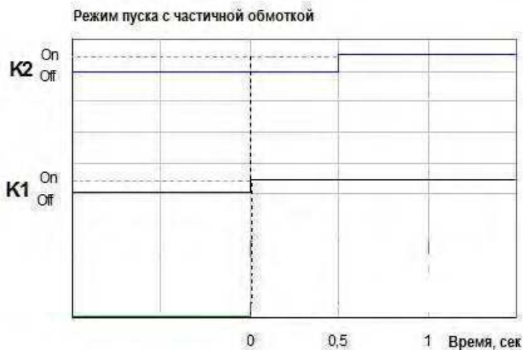
Рисунок 5-3 (с) Схематическая диаграмма задержки контактора пуска частичной обмотки
