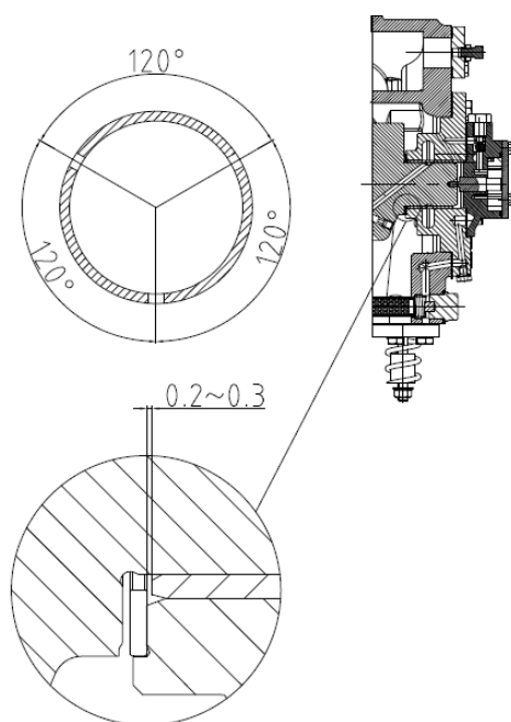
Рисунок 4-9 Схематическая диаграмма базовой втулки масляного насоса
