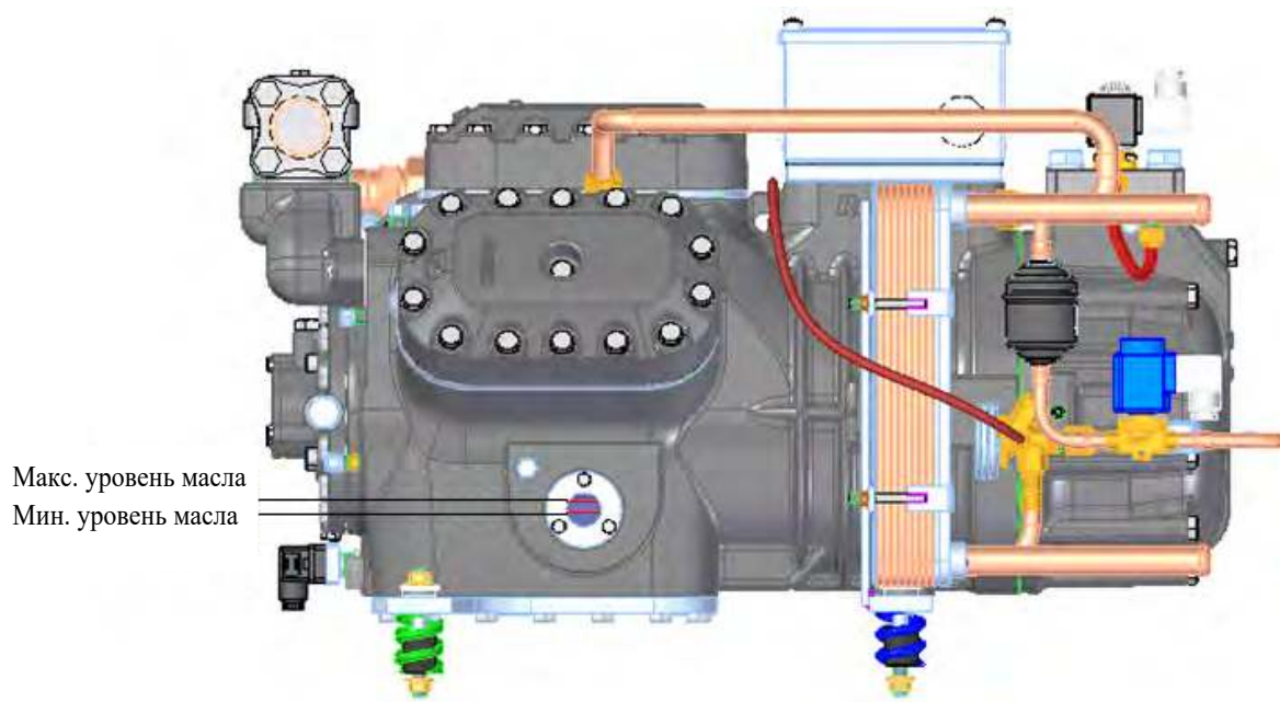
Рисунок 2-10 Маслосмотровое стекло
