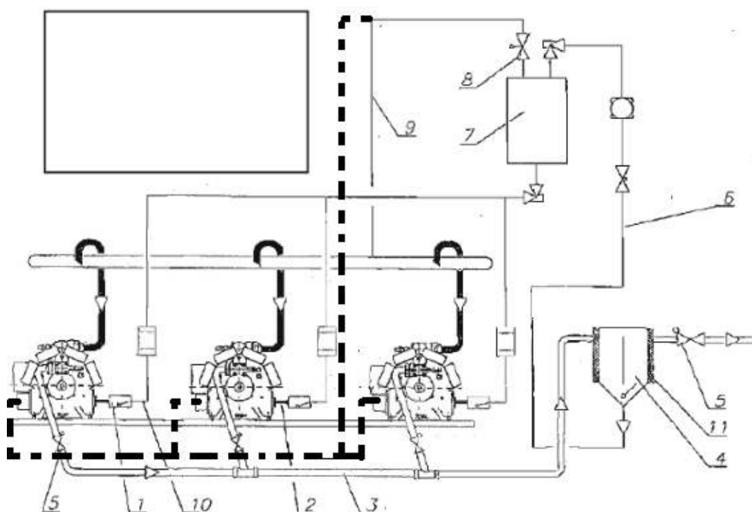
Рис. 12-1 Параллельное соединение с регуляторами уровня масла и одним маслоотделителем
