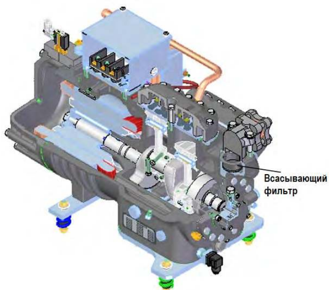
Рисунок 4-2 Расположение всасывающего фильтра серии SB6C
