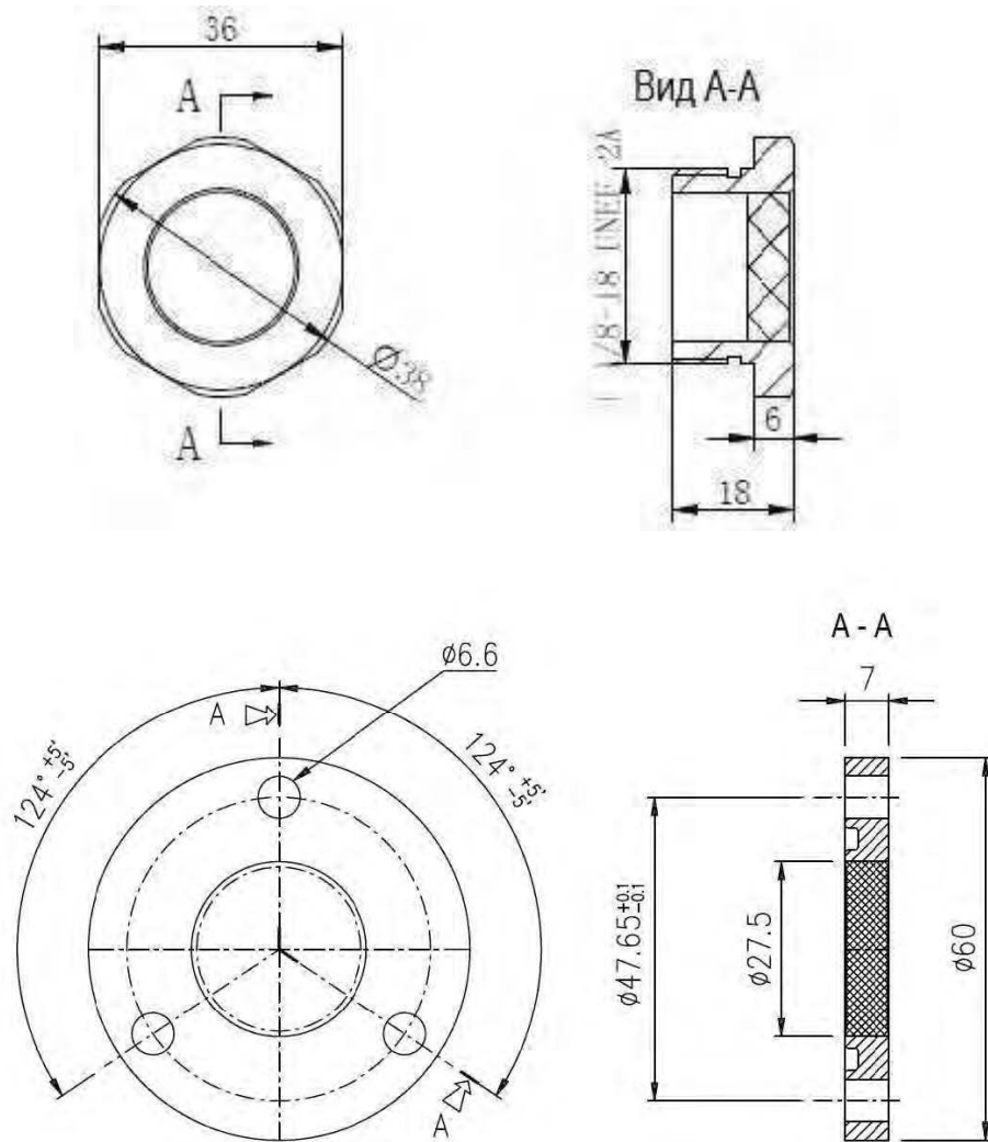
Рисунок 2-11 Габаритный чертеж маслосмотрового стекла
