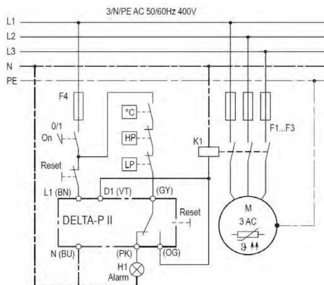
Рисунок 2-15 Схема подключения электронного реле перепада давления масла
