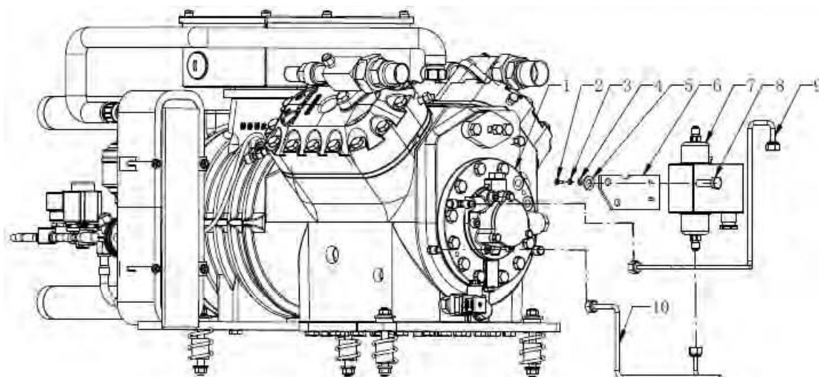
Рисунок 2-19 Компоненты механического регулятора перепада давления масла MP54 (код: 303191)
