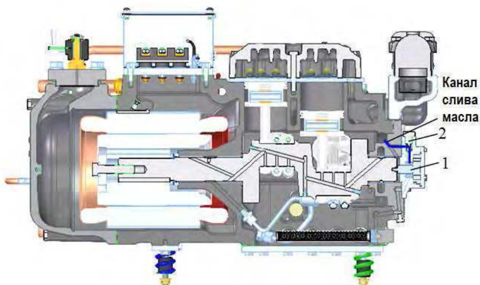
Рисунок 2-3 Масляный предохранительный клапан серии SBC
