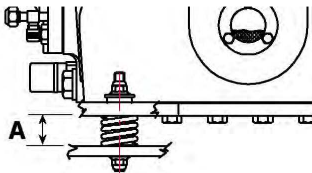
Рисунок 11-2 Пружинный амортизатор
