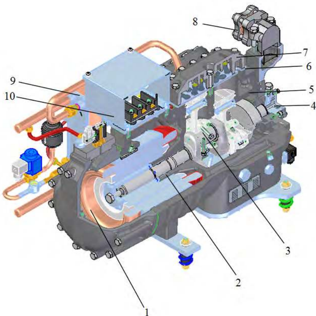
Рисунок 1-1 Структурная схема основных компонентов серии SBC
